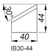
30°-os belső ferdevágó szerszám Magasság: 44 mm [IB30/44] Termékkód: NOZ-000023
