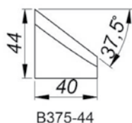
37,5°-os ferdevágó szerszám Magasság: 44 mm [B375/44] Termékkód: NOZ-000020
