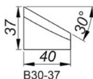
30°-os ferdevágó szerszám Magasság: 37 mm [B30/37] Termékkód: NOZ-000019
