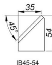
45°-os belső ferdevágó szerszám Magasság: 54 mm [IB45/54] Termékkód: NOZ-000026
