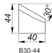
30°-os ferdevágó szerszám Magasság: 44 mm [B30/44] Termékkód: NOZ-000018
