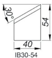
30°-os belső ferdevágó szerszám Magasság: 54 mm [IB30/54] Termékkód: NOZ-000025
