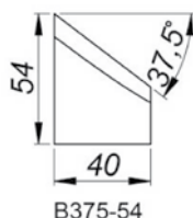
37,5°-os ferdevágó szerszám Magasság: 54 mm [B375/54] Termékkód: NOZ-000015
