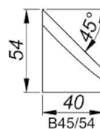
45°-os ferdevágó szerszám Magasság: 54 mm [B45/54] Termékkód: NOZ-000021
