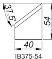
37,5°-os belső ferdevágó szerszám Magasság: 54 mm [IB375/54] Termékkód: NOZ-000024
